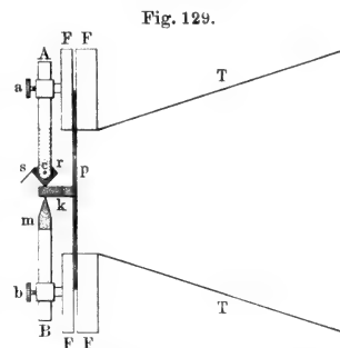
Apparat zur Projektion und Registrierung der Stimmenschwingungen, nach Samojloff.
